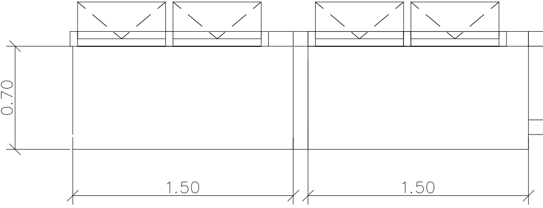
แปลนครุภัณฑ์ SS6 มาตราส่วน 1:25 (ล่างจาน-เก็บจาน ชั้น 1)
