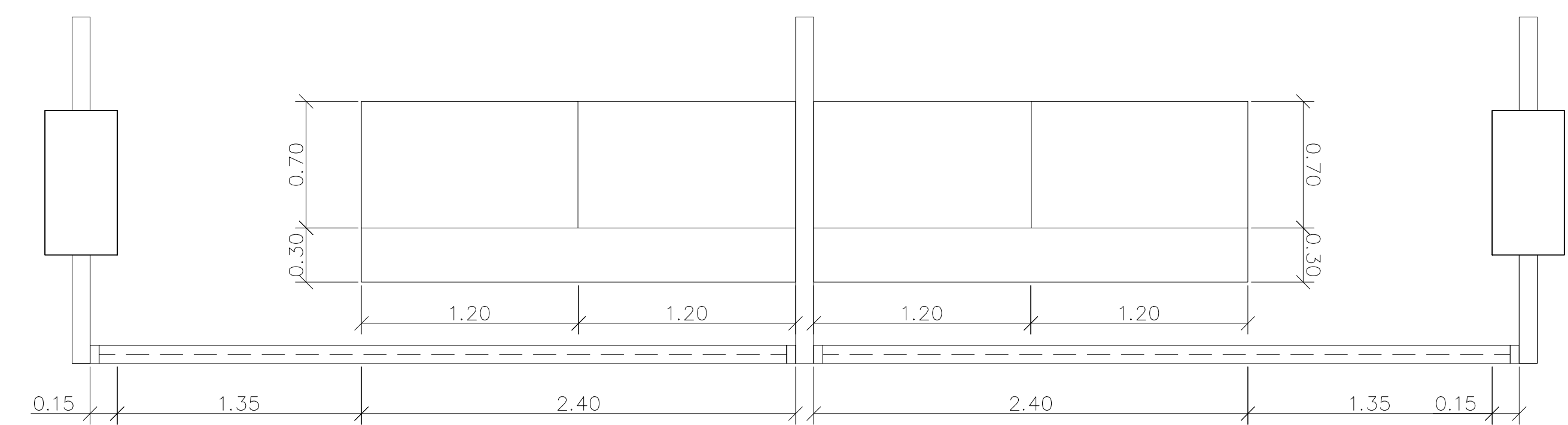
แปลนครุภัณฑ์ SS2.1 มาตราส่วน 1:25 (ร้านอาหาร 2,4,6,8 ชั้น 1)
