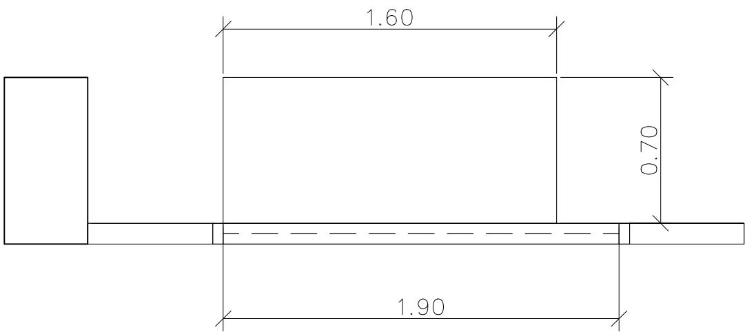
แปลนครุภัณฑ์ SS4 มาตราส่วน 1:25 (ล่างจาน-เก็บจาน ชั้น 1)
